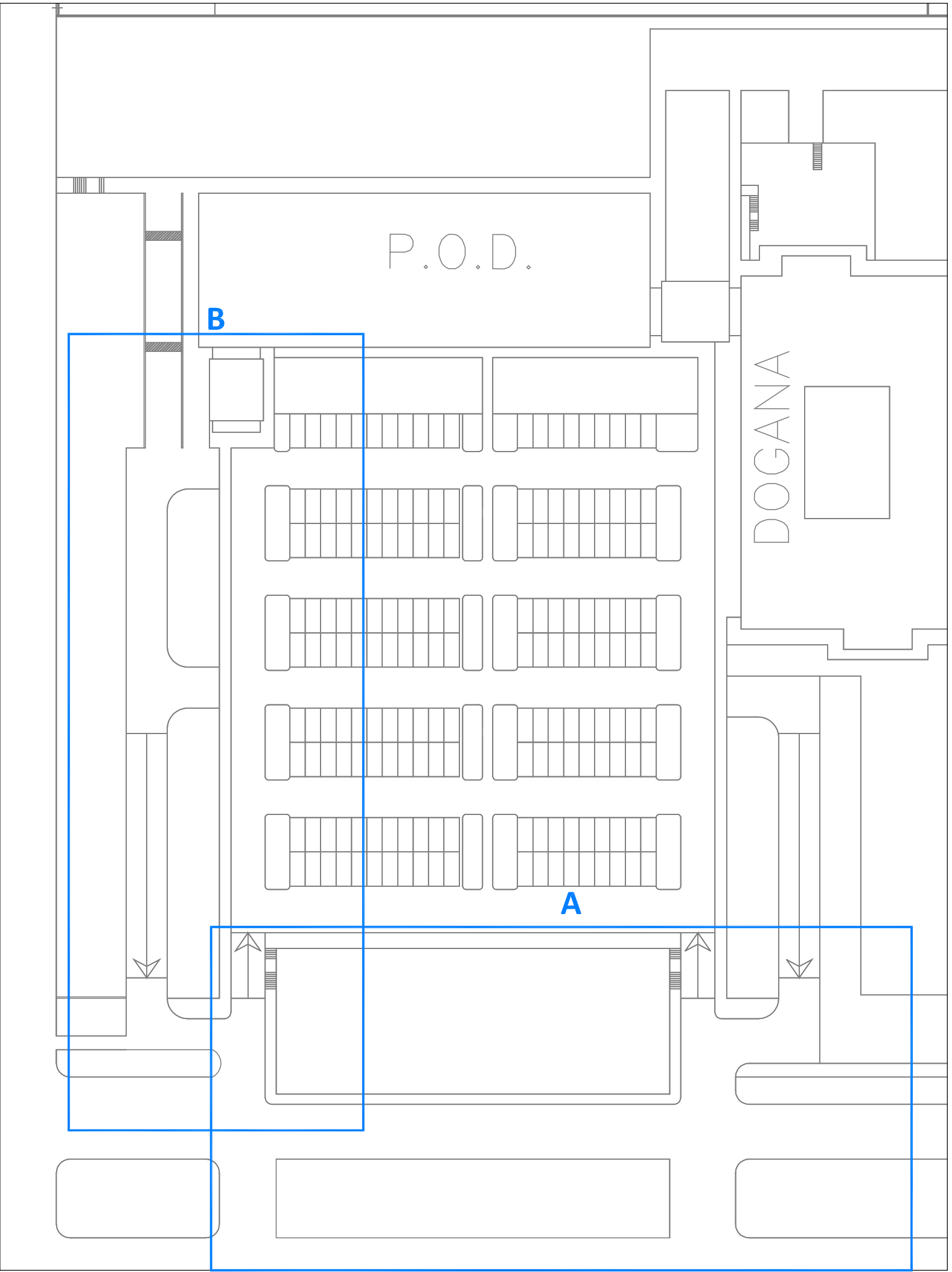
FASE LAVORATIVA (PIANO INTERRATO) ADEGUAMENTO CABINA MT/BT - SCALA 1:100
