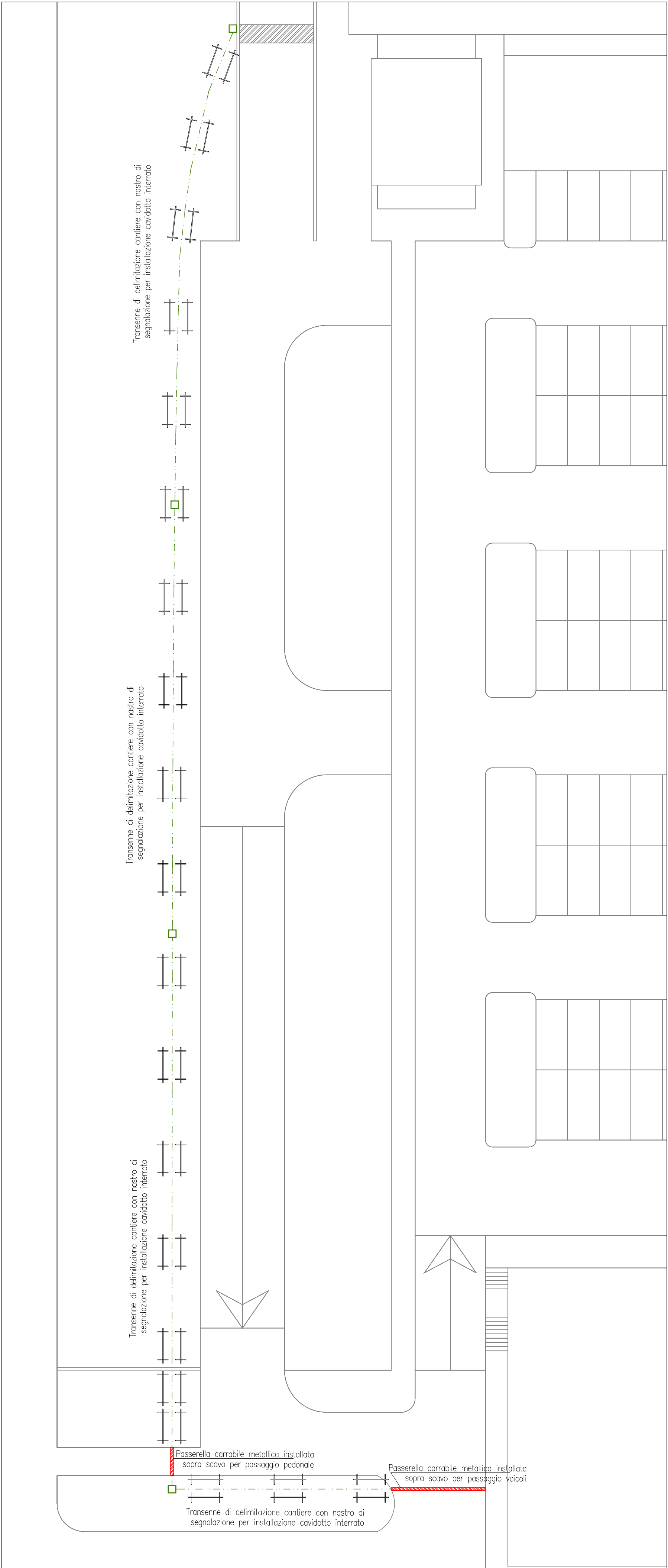
FASE LAVORATIVA (PIANO INTERRATO) ADEGUAMENTO CABINA MT/BT - SCALA 1:100
